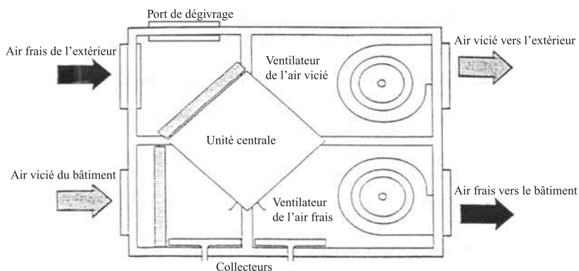
Figure 1 Modèle 1100 VUE AVANT
